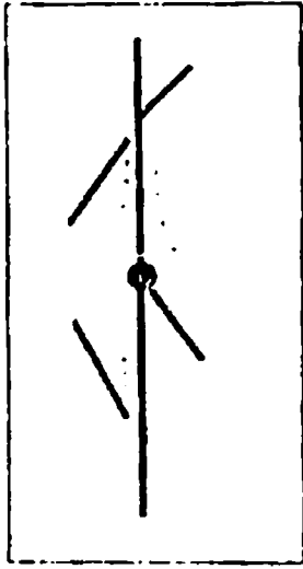
موقع الشمس في المجرة
